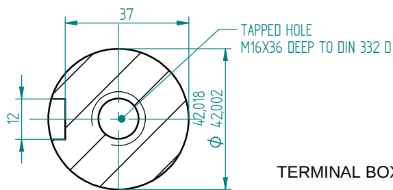
Przekrój A-A 1:1
